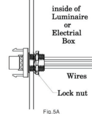
Fig.5A
